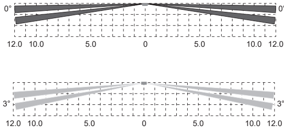
BXS-AM – Vista desde arriba
