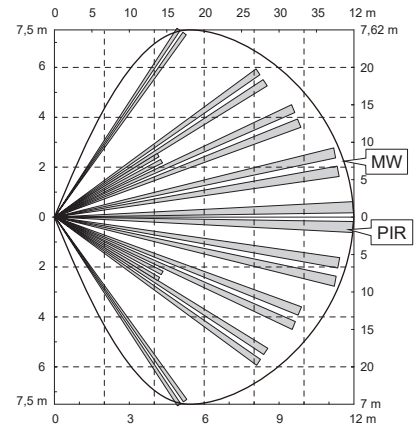
QXI-DT – Vista desde arriba
